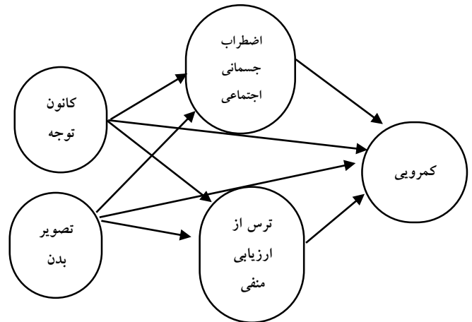
شکل ۱: دیاگرام مسیر مربوط به مدل مفهومی
